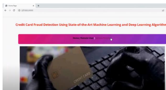
Fig.2. Login page.
